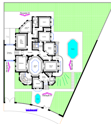
Térreo A = 332,47 m 2
